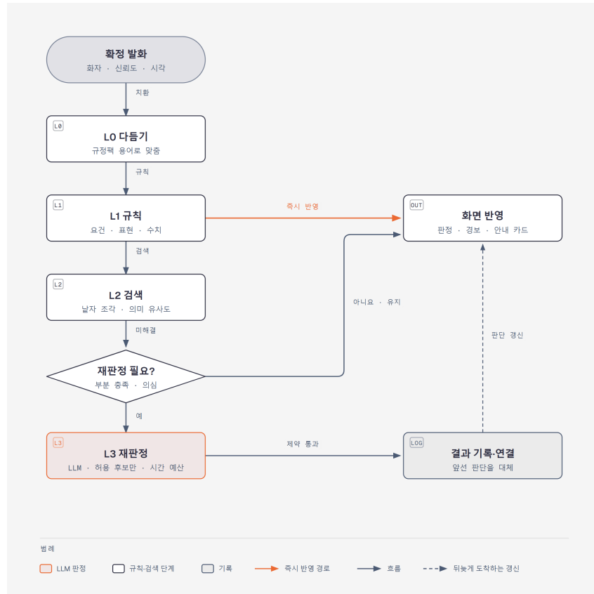
도식 3. 엔진 담당자의 설계를 바탕으로 재구성한 단계별 판정 흐름.
