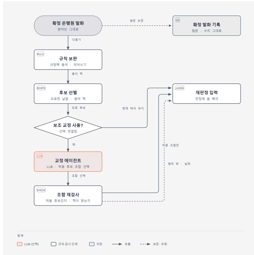
도식 4. 규칙으로 하는 용어 보완과, 선택으로 켜는 언어 모델 보조 교정의 경계.
