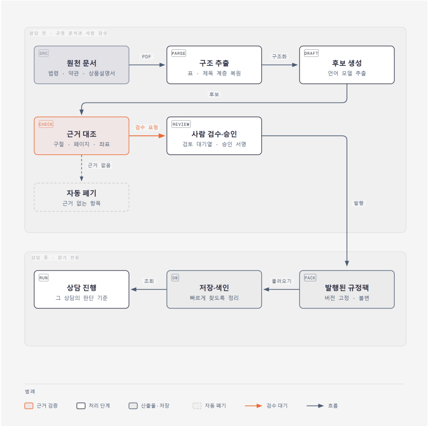
도식 5. 상담 전에 미리 하는 규정팩 구축과, 상담 중에는 읽기만 하는 발행물의 경계.
